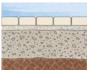
Fig. 15 detaje të shtrimit të ambienteve të jashtme me pllaka guri
