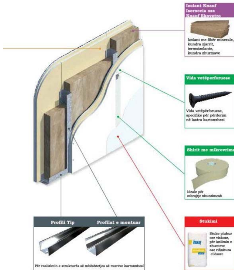
Fig. 9 detaje te montimit te kartonxhesit
